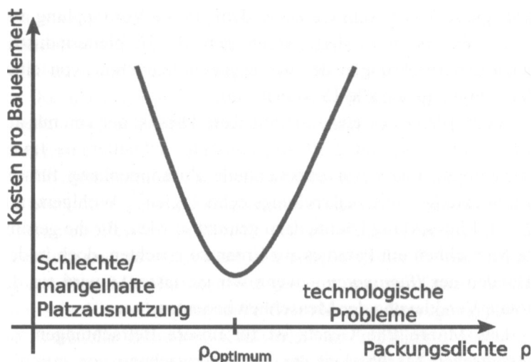
Abb. 1.11.1: Kosten pro Bauelement eines integrierten Schaltkreises als Funktion der Anzahl der Bauelemente pro Flächeneinheit (Packungsdichte)
